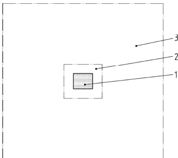
Рисунок 1 – Расположение зон непосредственного окружения и периферии по отношению к зоне зрительной задачи
