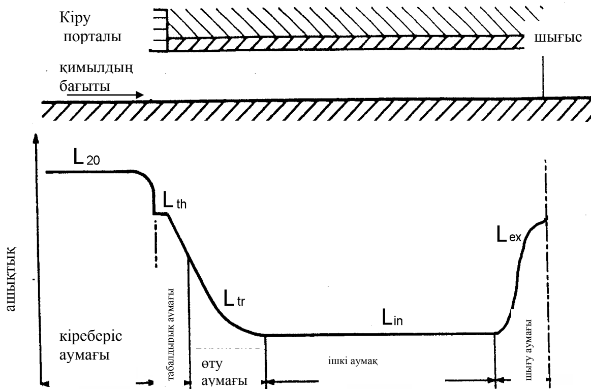
Д 1 сурет – Күндізгі тәртіптегі туннельдің жарық аймақтары
