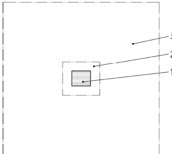
1 сурет – Ең кіші габариттер мен тікелей қоршау өңірлерінің және шет өңірлердің (периферияның) көру есебі өңіріне қатысты орналасуы 1 – көру есебінің өңірі; 2 – тікелей қоршау өңірі (ені 0,5м кем емес аралық); 3 – периферия өңірі (орынжай ішіндегі ені 3м астам аралық)
