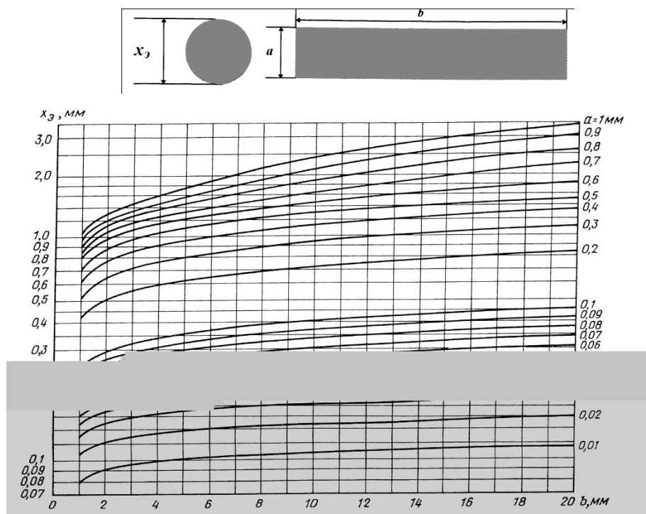
Б 1-сурет – Көзден нысанға дейін 500 мм-ге дейінгі қашықтық кезінде созылыққы айыру нысандарының эквивалентті мөлшерін айқындауға арналған номограмма
