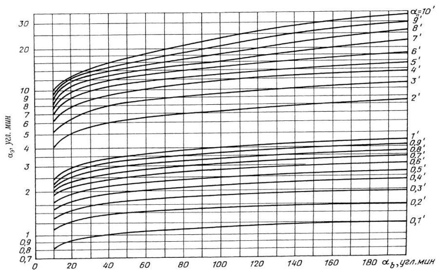
Б 2-сурет – Көзден нысанға дейін 500 мм асатын қашықтық кезінде созылыққы айыру нысандарының эквивалентті мөлшерін айқындауға арналған номограмма
